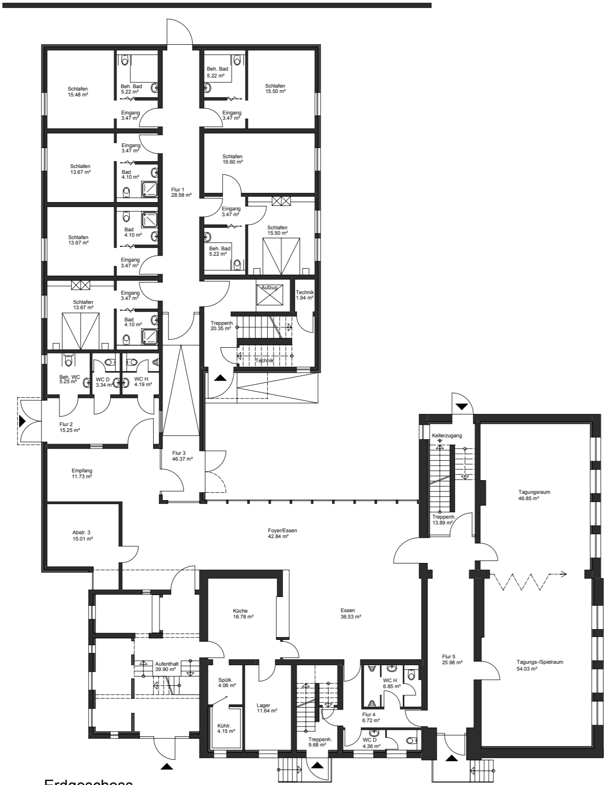
Erdgeschoss
