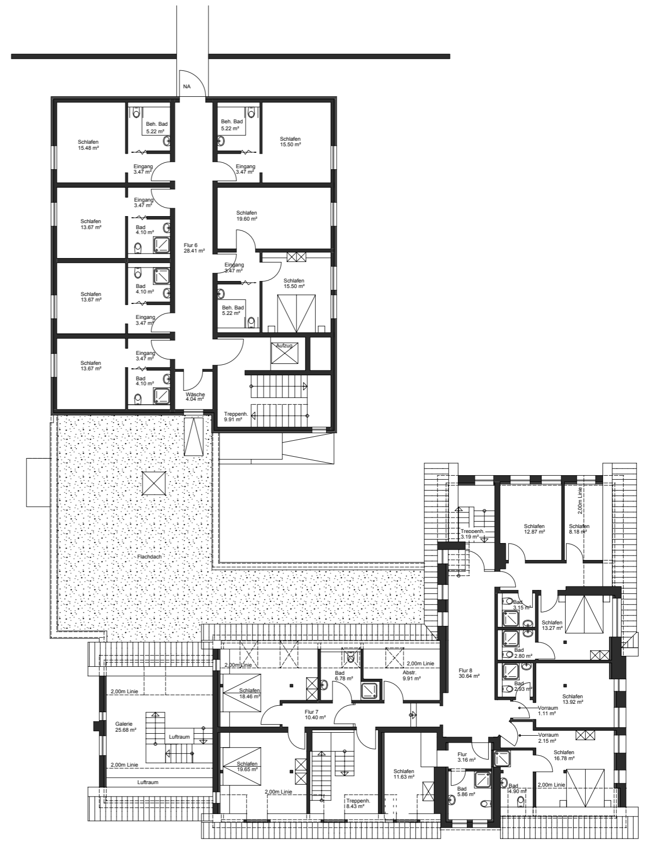
Obergeschoss
